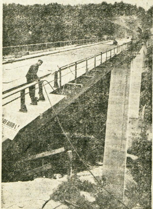
Most čez Peračico pri Lancovem je zadnji trd oreh, da bi odprli novo avtomobilsko cesto od Bistrice do Podvina. Most je širok 10 in dolg 370 metrov in bo sposoben za najtežji promet. Do avgusta upajo da bodo vložili še manjkajoče železne konstrukcije v dolžini 100 metrov in odprli promet. Mnogi vozniki si tega zelo želijo
