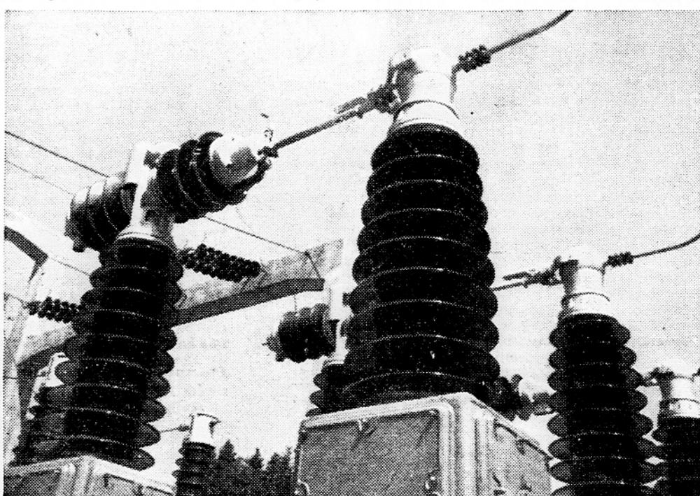
Poleg nove hidrocentrale v Medvodah montirajo 110.000 voltno prostozračno transformatorsko postajo
