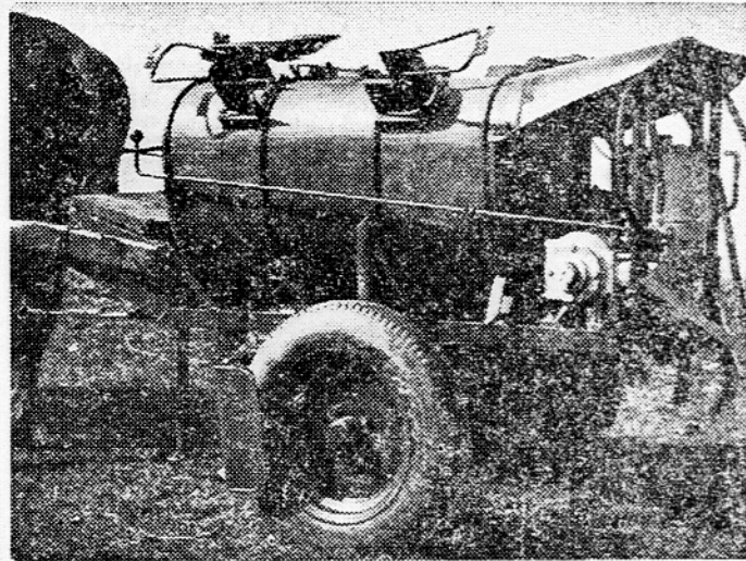
Motorna sadna škroplilnica
