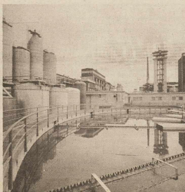
Star betonski kislinski stolp je s pridobitvijo novih naprav za regeneracijo kisline prenehal z obratovanjem
