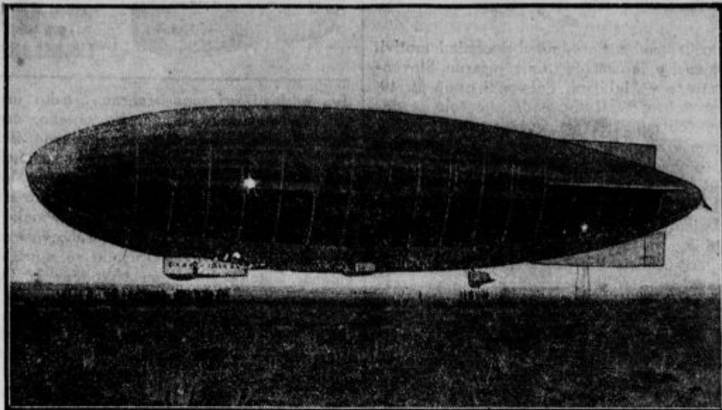
Nobilov zrakoplov »Italia«,
