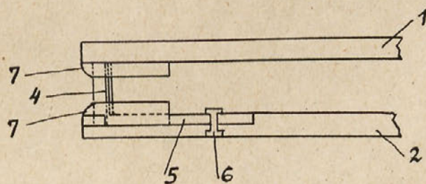
Slika III. Presjek A-B
