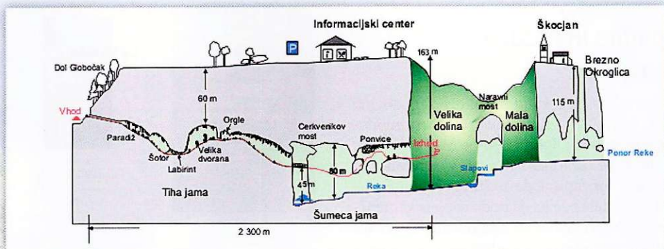
Prečni prerez Škocjanskih jam
