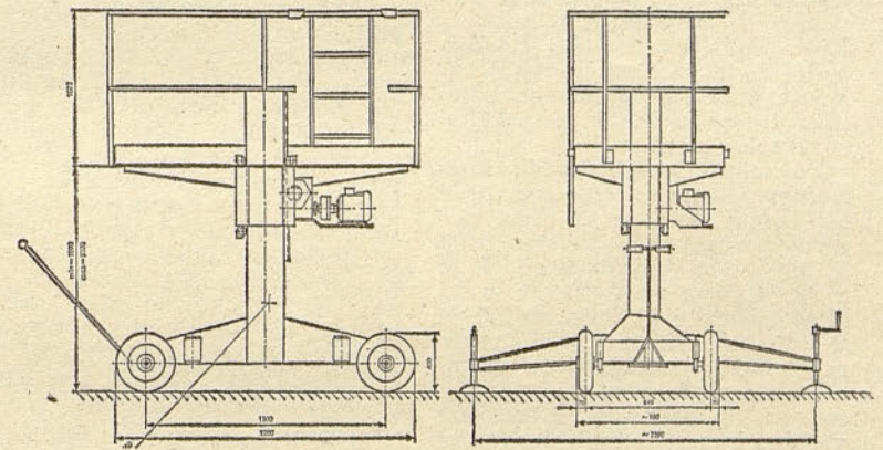
Delovni oder FM 1000/1S skica
