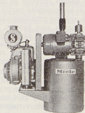
Miele — molzne naprave, agregat LM 130 z bencinskim motorjem za dva molznjaka
