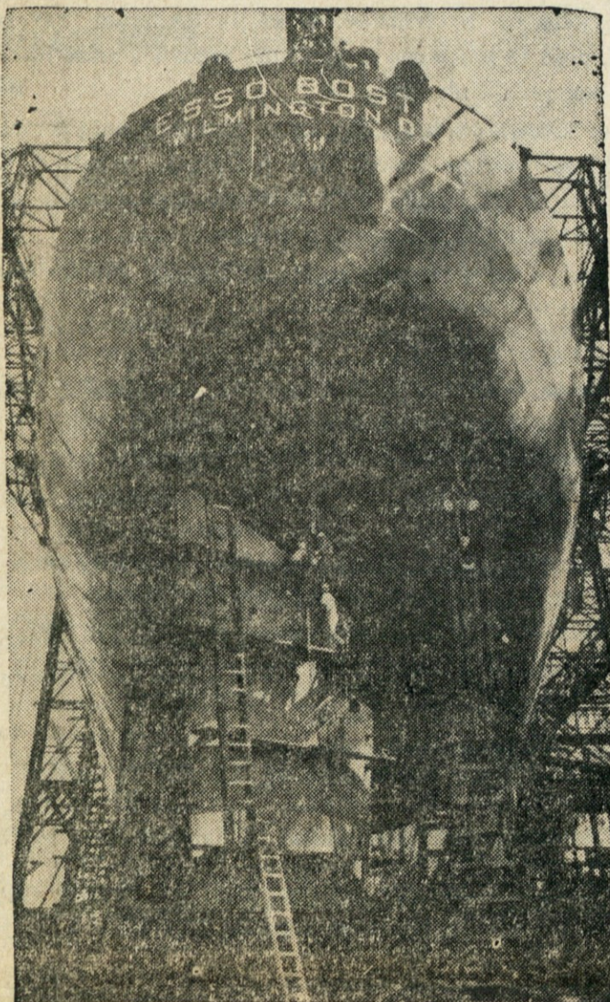
VELIKANSKO KRMILLO — Na sliki vidimo delavce, ko pritrjujejo 85.000 funtov težko krmilo na novo petrolejsko ladjo "Esso Boston" v Newport News, Va. Nova ladja je dolga 740 čevljev in bo sprejela vase do 17 in pol milijona galonov olja.
