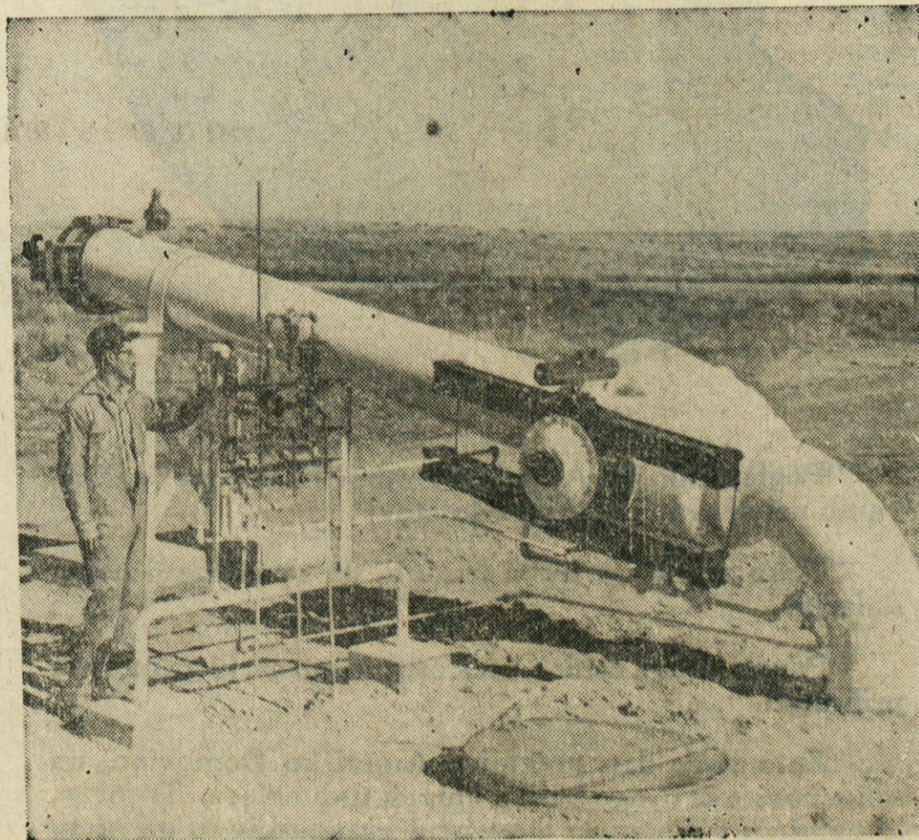
TOP? — Naprava na sliki je podobna topu in v resnici strelja posebne neoprenske krogle po cevovodih za plin, da jih očisti za nemoten tok plina. Naprava stoji v bližini Mocane, Okla.
