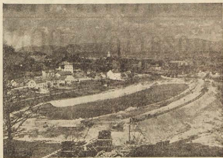
Celje — Regulacijsko področje Savinje. Gradbena dela hitro napredujejo. Prvi železniški most, provizorijski je že zgrajen. Na sliki desno je železniška proga, speljana po novem nasipu do drugega provizorijskega (ki ga še gradijo). Predvidevajo, da se bo železniški promet po novem odcepu začel konec junija. Takrat bodo lahko odstranili oba stara železniška mostova in prekopali mrtev rovak Savinje
