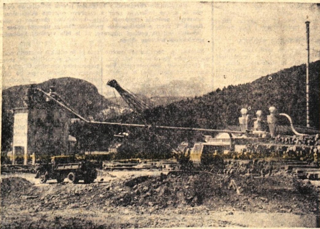
Zamisel in osnovni koncept mehanizacije in funkcionalne ureditve krišča — prostora za skladišče hlobovine so programsko izdelali na LIP-u Bled, končni projekt pa: Projektni biro za lesno industrijo LRS v Ljubljani. Na sliki: Zemeljska dela za ureditev mehaniziranega krišča na bazenskem obratu »Tomaž Godec« v Bohinjski Bistrici norm alno potekajo. Če bo ugodno vreme bodo končana predvidoma v enem mesecu
