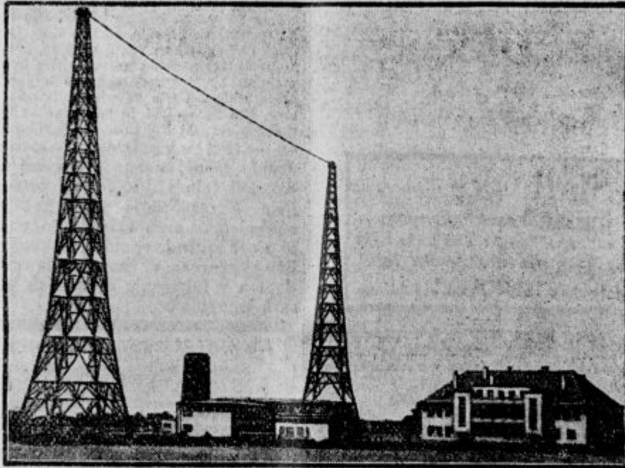
Največja radijska oddajna postaja v Evropi. Pred kratkim so končali z graditvijo nove radijske oddajne postaje-velikanke v Lipskem. Antenska energija postaje znaša 150 kilovatov in je radi tega postaja najmočnejša v srednji in zahodni Evropi.
