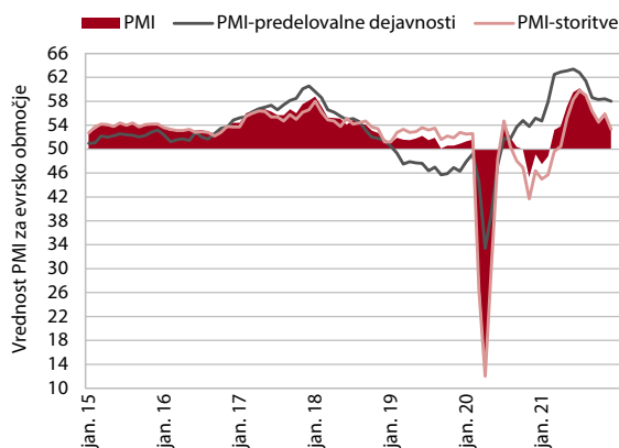
Slika 1: Sestavljeni kazalnik vodij nabave, PMI, za evrsko območje
