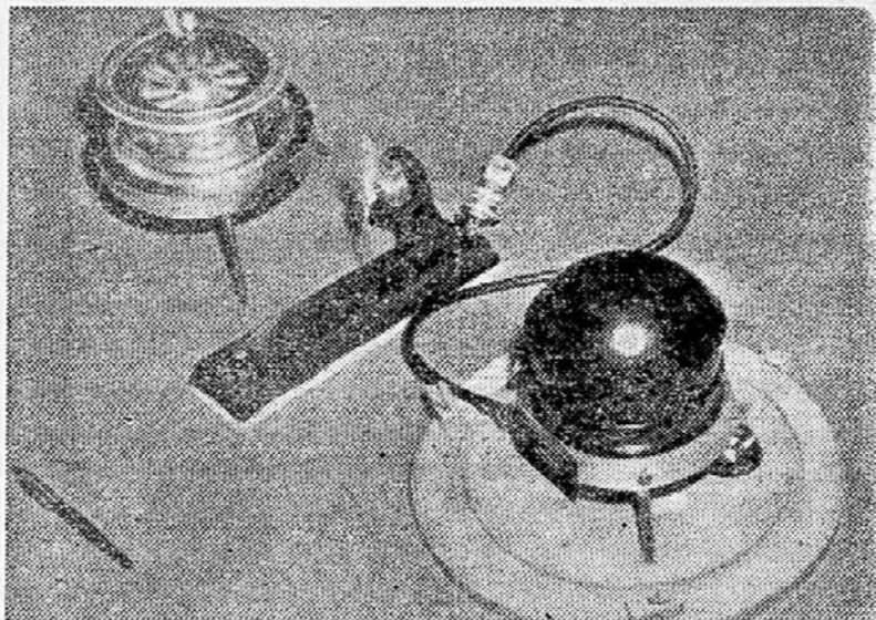
V ZDA so izdelali najmanjši termoelektrični generator, ki dobi energijo od radioizotopov. Baje je dvajsetkrat manjši od vseh do sedaj znanih generatorjev, ki pretvarjajo toplotno energijo v elektriko. Ker so generatorji izredno majhni in lahki, jih bodo uporabljali v medcelinskih in medplanetarnih raketah za radijske oddajnike. Da si laže zamislimo, kako veliki so novi generatorji, leži v levem spodnjem kotu posnetka nalivno pero.
