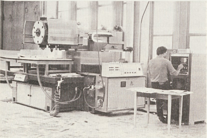
Delček sodobnosti — obdelava lesa na CNC rezkarju
