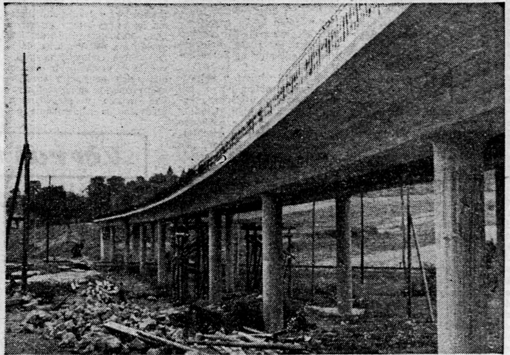
Avtocesta Ljubljana-Zagreb, odsek (Ivančna gorica) viadukt čez staro cesto in železnico
