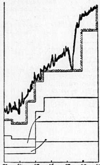
Primer obratovanja glavne akumulacijske elektrarne na frekvenco in premostitve defekta enega agregata pretočne elektrarne; valovite črte so obtebe različnih elektrarn, črtkani del pa obteba akumulacijske elektrarne, nazobčana krivulja pa dejanski diagram potrošnje.
