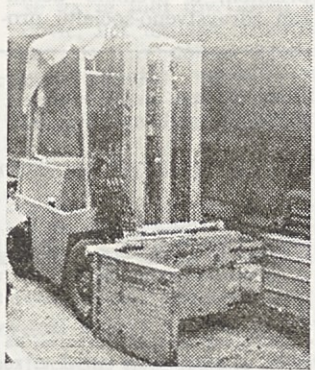
Viličar s hidravličnimi kleščami za bale bombaža, zaboje ali drugo blago v večjih kosih
