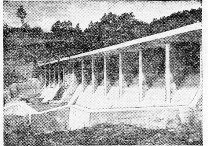
Hidromehanične naprave dolinske pregrade za hidrocentralo Vinodol.
