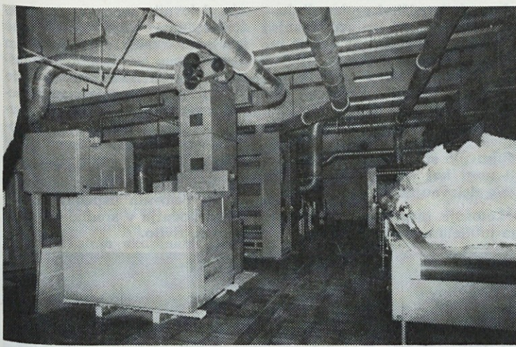
Stroja — MTO (Micro Tuft Opener) v ospredju, namenjen za fino odpiranje kosmičev ob istočasnem čiščenju in izločanju manjših trših delcev nečistoč, in v ozadju, večji stroj, odstranjevalec prahu DR (Dust Renover) odstranjuje mikro prah s pomočjo koncentriranega pretoka zraka
