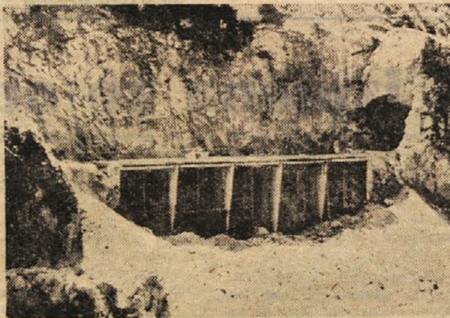
Na Zasavski cesti je vsak dan kaj novega. Nov most med predoroma v Tolmunih zdaj že dobiva končno obliko. Na sliki: del novega mostu, ki ga gradi Gradbeno podjetje Litija
