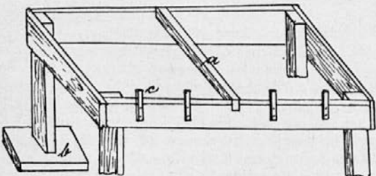
Leseno ogrodje tople, ozir. mrzle grede. a opora za okvir, b podloga pod nogo, c opore, ki zadržujejo okna, da ne drse
