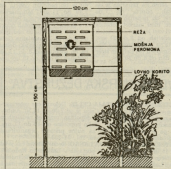
Montaža ploščate režaste pasti znamke Theysohn.
