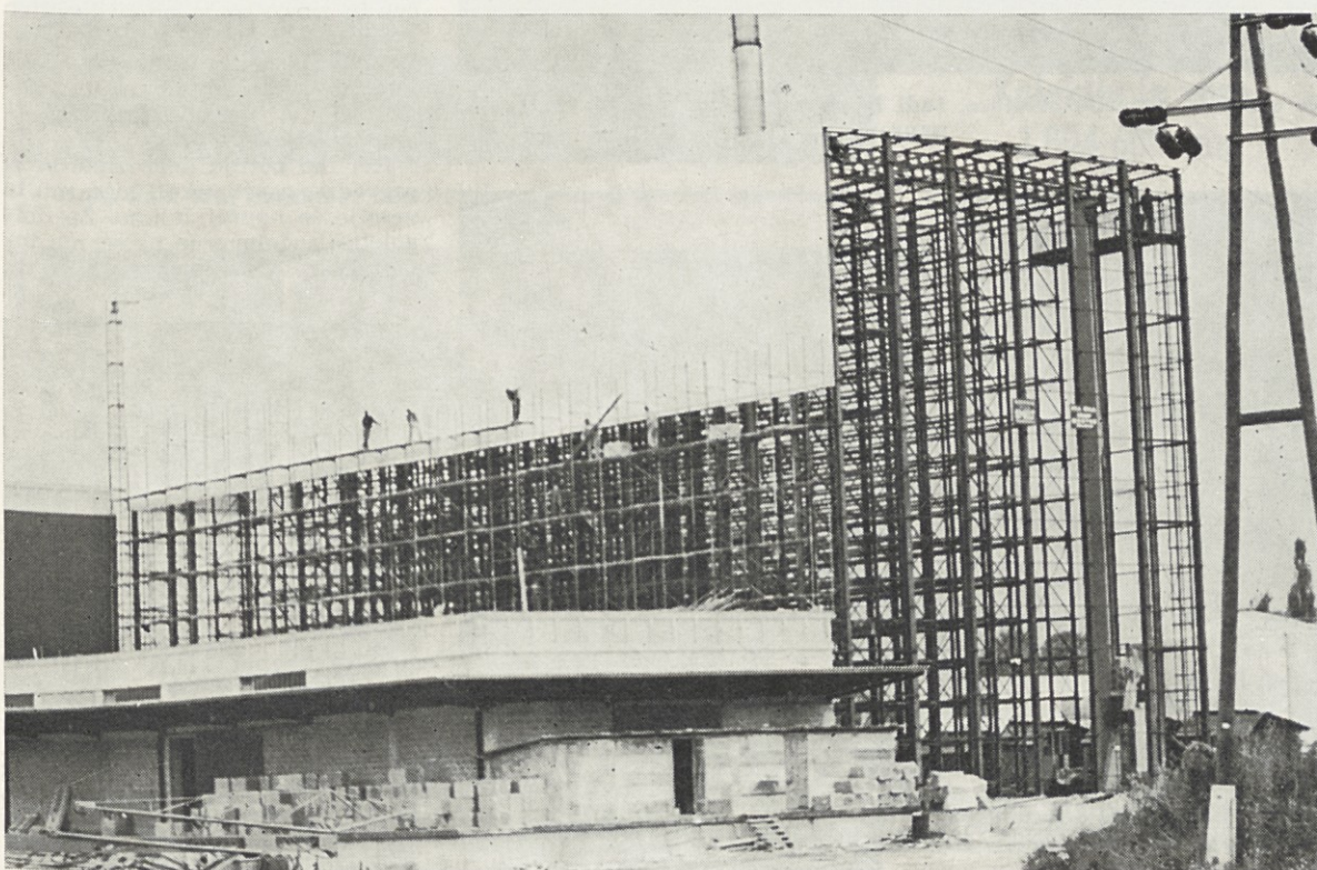
3. 9. 1976 so visoko regalno skladišče začeli oblagati s stenami. Same regale in ogradje pa je bilo treba postaviti že prej ob zgradbi V. PS (Foto: Edvard Anžur)
