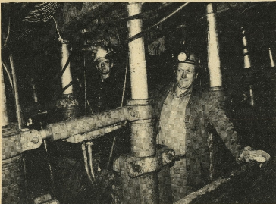
Nadzornik Emil Koncilja in kopač Martin Brečko na odkopnem čelu s SHP podporjem v jami Rudnika Trbovlje.
