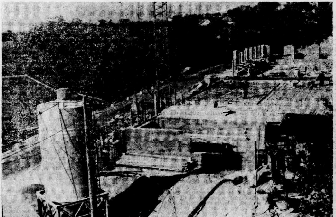
REMIZA ZA PODZEMELJSKO ŽELEZNICO — V Postojnski jami so začeli prvo fazo gradnje nove krožne proge. Levo od sedanjega vhoda bo trinadstropna remiza (na sliki), v kateri bodo tudi mehanična delavnica in skladišča. Ko bo stekla krožna proga, bodo k sedanjim dvem kompozicijskim dopili še eno, tako da se bo lahko hkrati peljalo skozi jamo 360 ljudi. Foto: Selhaus
