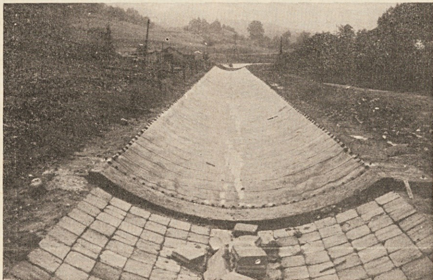
Del izgotovljene nove struge potoka Katredežca v Zagorju. Na jalovinski podlagi so položeni betonski kvadri, po površini teh kvadrov pa je položena gumijasta ponjava.
