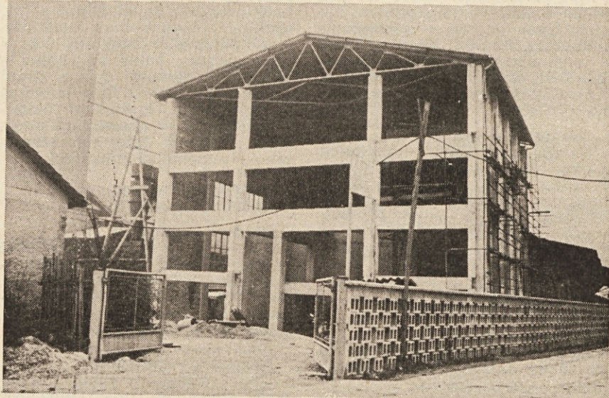
Gradnja tovarne na opekarni v Trbovljah. Posnetek je od 17. novembra 1970. Foto: Inž. Tone Bregant
