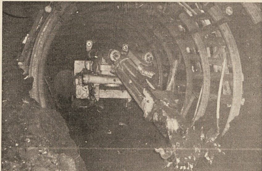
Stroj za izdelavo jamskih prog F 6-A pri delu v polju Polaj II na rudniku Trbovlje. Rudarji ga imenujejo po domače »štreakenhajer«.
