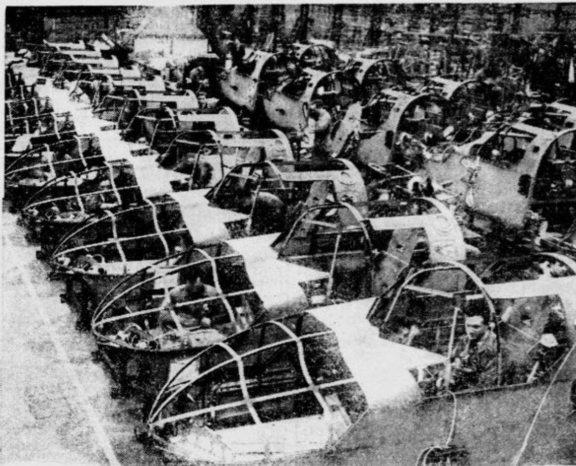
Ena največjih tovarn letal na svetu, ki se nahaja »nekje« v Angliji. V tovarni je zaposlenih nekaj tisoč delavcev, ki noč in dan izdelujejo bombnike
