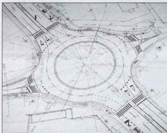
Projekt krožišča na klancu
