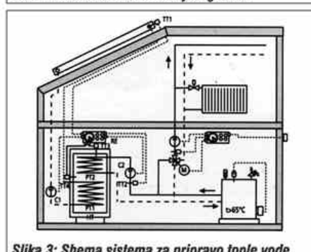
Slika 3: Shema sistema za pripravo tople vode
