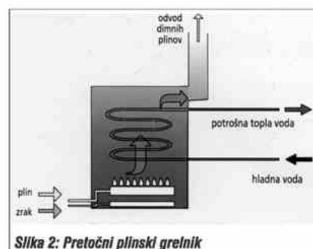
Slika 2: Pretočni plinski grelnik
