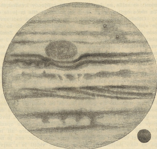
Jupiter v razmerju do naše Zemlje, ki je na naši sliki na desni strani spodaj
