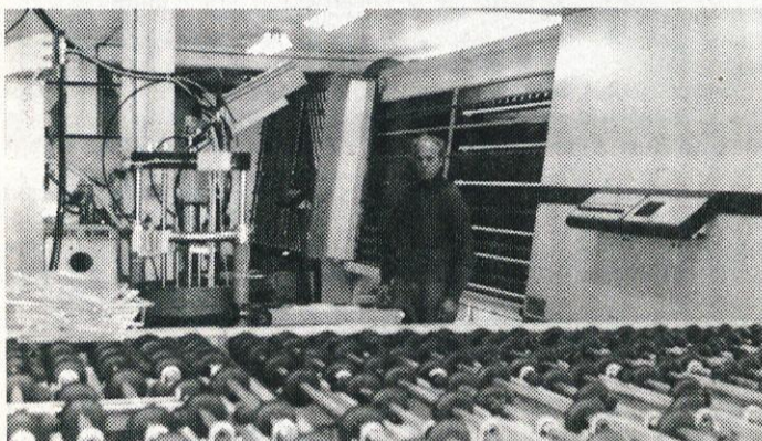
V steklarstvu Volčini – VITRAM na Viru so v petek, 12. novembra, predstavili najbolj sodoben steklarski stroj – steklarsko linijo za izdelovanje termopan stekla. Napravo so uvozili iz Italije
