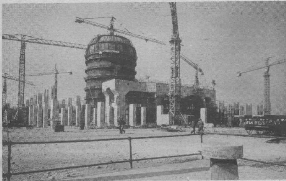
Po vrsti hidro in termo elektrarn je Gradis prevzel tudi gradnjo prve jugoslovanske jedrske elektrarne v Krškem
