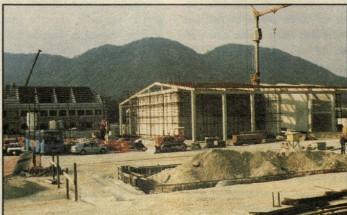
Pogled na bodočo avtocestno vzdrževalno bazo
