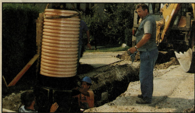
Izgradnja primarnega kanalizacijskega voda v Dolenji vasi
