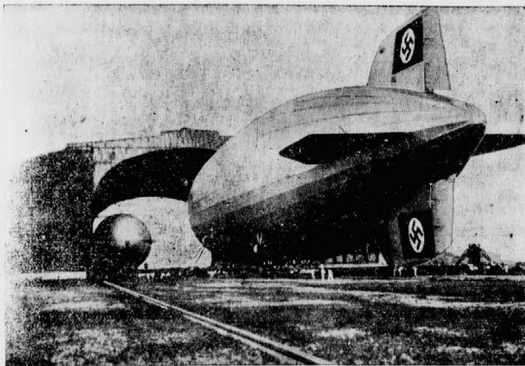
Bei der letzten Landung des Luftschiffes „Hindenburg“ in Amerika wurde der Lufttrieb in die Luftschiffhalle von Lakehurst gebracht. Zu diesem Zweck mußte das amerikanische Luftschiff „Los Angeles“, das als „ZR 3“ ebenfalls in Friedlandshafen gebaut ist, beiseitegerückt werden, um dem „Hindenburg“ Platz zu machen. Wie klein sieht die „Los Angeles“ neben dem „Hindenburg“ aus! (Presse-Bild-Zentrale-M.)
