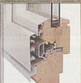
Leseno okno Plus
