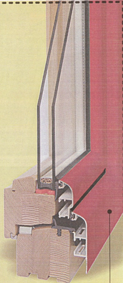
Les-aluminij SOFT okno
