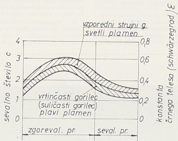
Diagram 2: faktor ε in sevalno število c zemeljskega plina v odvisnosti od zgorevalne poti
