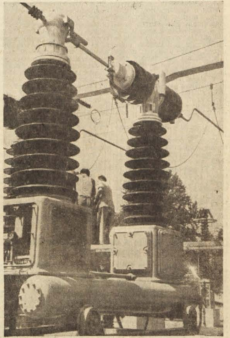
Del transformatorskih naprav hidrocentrale Medvode
