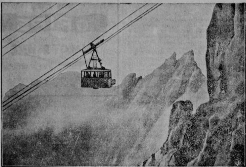
Železnica na Zugspitze (2964 metrov), ki so jo po velikih tehničnih težkocah sedaj srečno dovršili.
