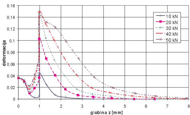
Slika 6: Plastični raztezki Figure 6: Plastic strain
