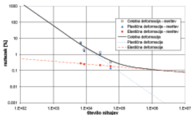
Slika 1: Wöhlerjeva krivulja za normalizirano jeklo C45
