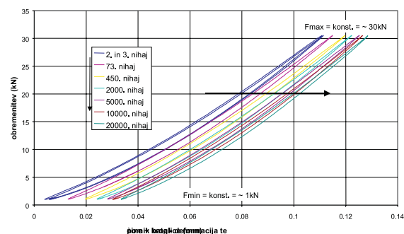
Slika 3: Diagram obremenjevanja (rast deformacije) za F_{MAX} = 30kN
