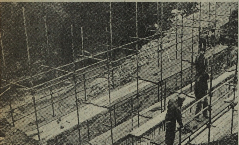
Pred mesecem dni smo pričeli graditi most čez Kokro. Narejen bo iz največjega prostoležečega prednapetega nosilca v Jugoslaviji, dolgega 50 m
