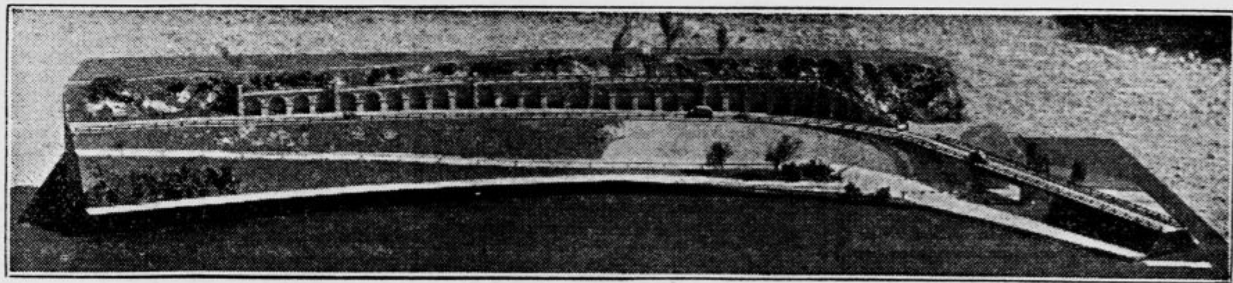
Z razstave »Cesta«: model nove državne ceste s mogočnimi opornimi stebri in nadvozom čez železniško progo pri Kranju —
