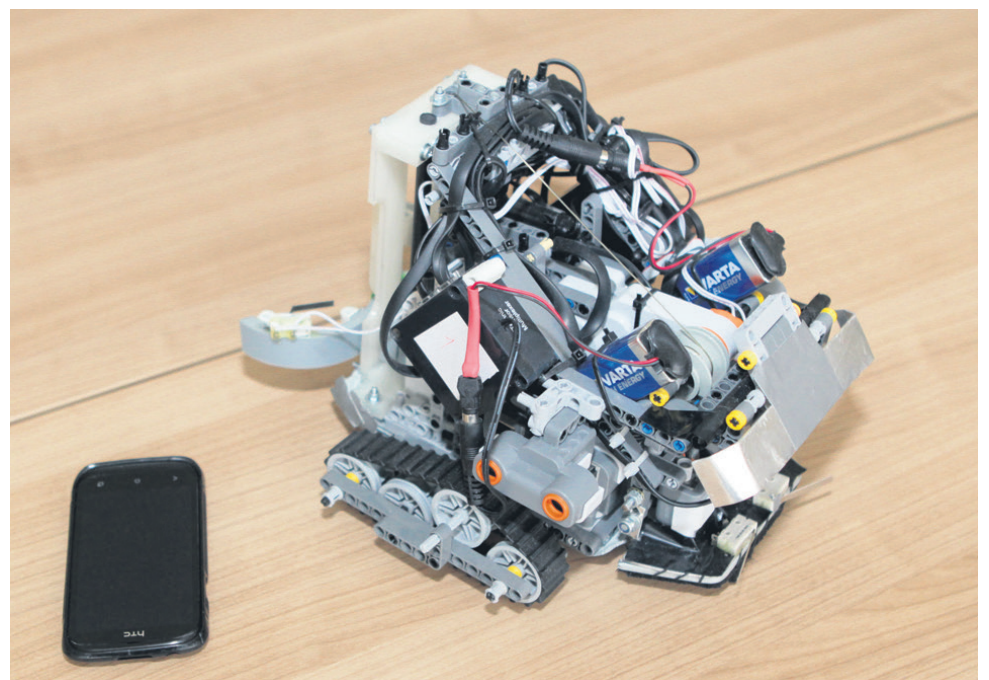
Izdelek skupine Triple-J, robot, s katerim so se pomerili na svetovnem tekmovanju v Braziliji.
