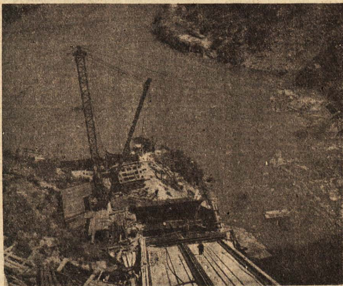
Kakor smo že poročali, so v Jablanici zaprli jez in v kotlini Neretve je začelo nastajati jezero. Del jezera, ki nastaja, vidimo na sliki
