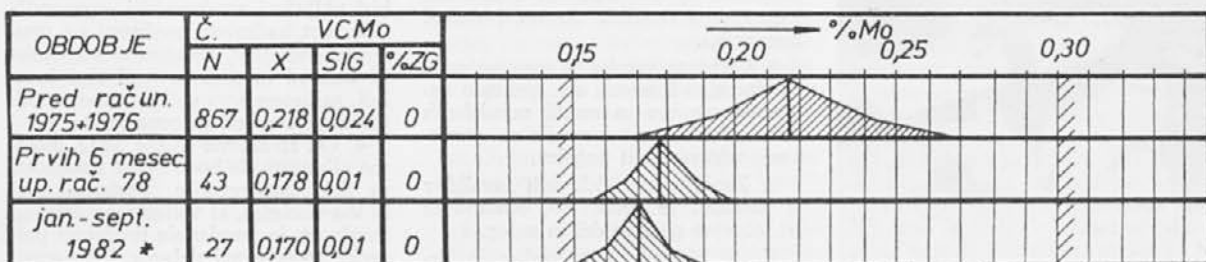
Slika 4: Tipično znižanje vsebnosti molibdena v jeklih VCMo
