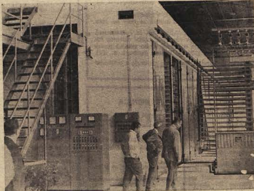
Največja pridobitev ljubljanskih opekar v obratu OPEKA so velike umetne sušilnice in naprave za mehaniziran notranji transport.
