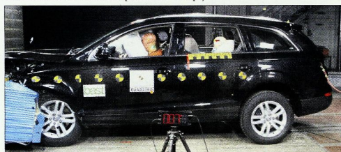
Audi Q7 med preskusnim trčenjem
