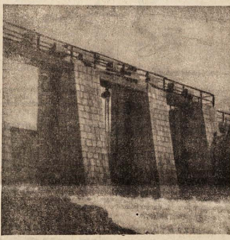
Zatvornica hidrocentrale na Zgornji Zeti v Črni gori
