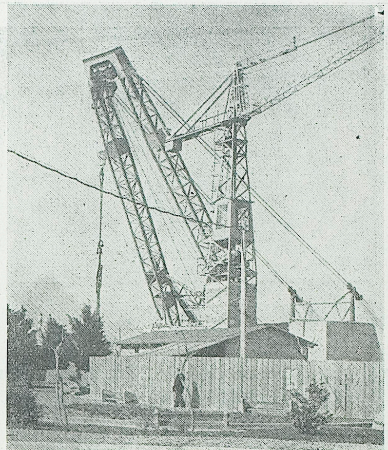
Nadaljevanje gradnje novega koprškega tovornega pristanišča lepo napreduje, hkrati pa se tudi promet razvija po načrtu. Naša slika posreduje prikazuje srečanje suhozemske in pomorske mehanizacije, ki sta udeleženi pri delih za novo pristanišče. Ko bo letos končana gradnja prve etape 400 m pristaniške obale, bodo lahko hkrati pristajale in manipulirale s tovorom po tri čezoceanske srednje tonaže, kar bo omogočilo že proti koncu tega leta izdatno povečanje prometa
