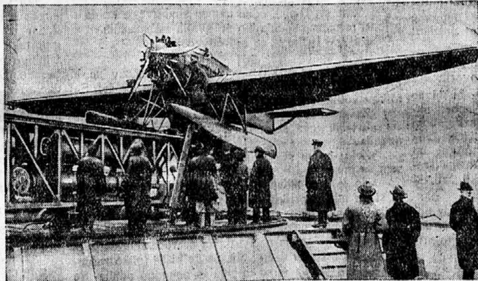
Za parnikom »Bremen« so Nemci zdaj opremili tudi parnik »Europo« s katapultnim letalom. Stroj je takozvan »Junkers-Metalltieflieger« tipa W 35. Levo v ospredju so vidne posode s stisnjenim zrakom, s katerega pomočjo izstrelijo letalo na odprtem morju.
